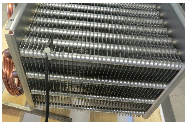
Plassering fordamperføler 1
