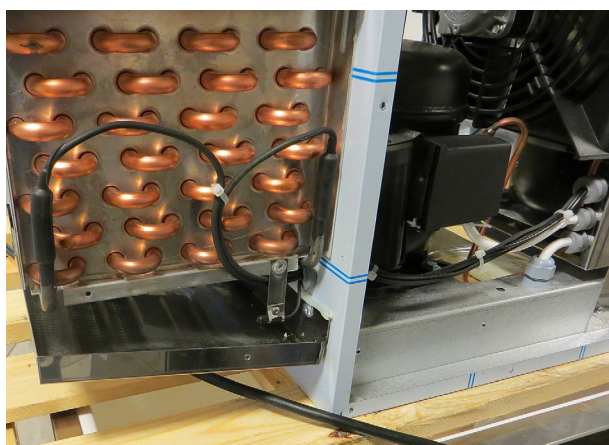
Plassering termostاتفøler
