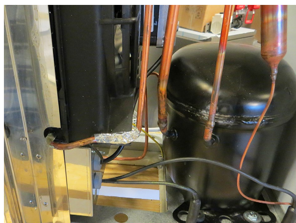
Plassering kondensatorføler
